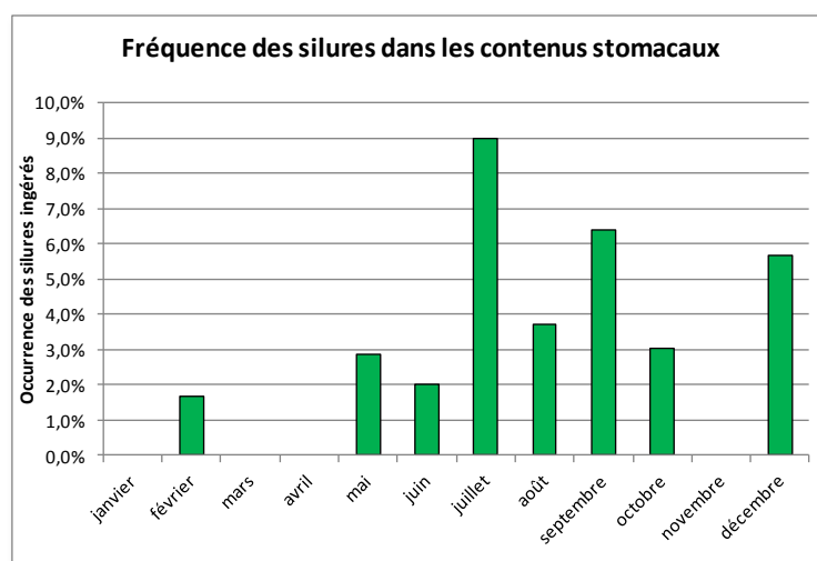
Figure 20 : fréquence des silures dans les contenus stomacaux
