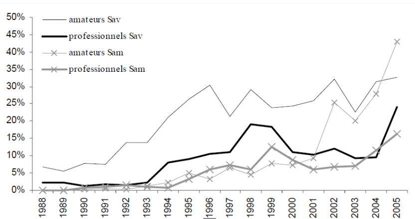
Figure 7: évolution de la part prise par le silure glane dans le total des captures des pêcheurs amateurs et professionnels de la Saône aval (Sav) et de la Saône amont (Sam) entre 1988 et 2005 (source : Valadou, 2007).
