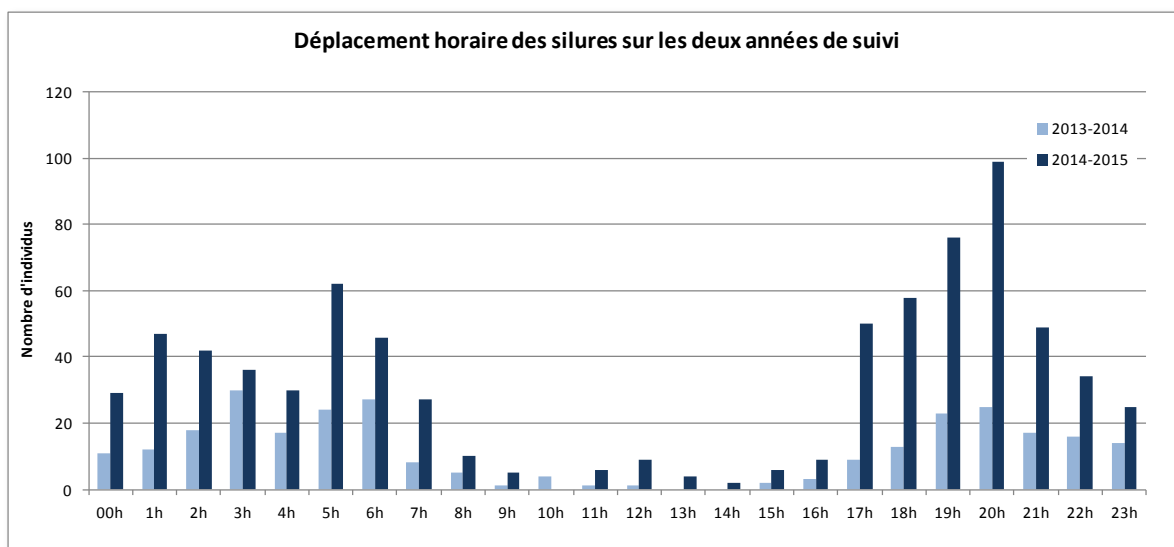
Figure 30 : activité journalière des silures observés à la station de vidéo-comptage de Jons
