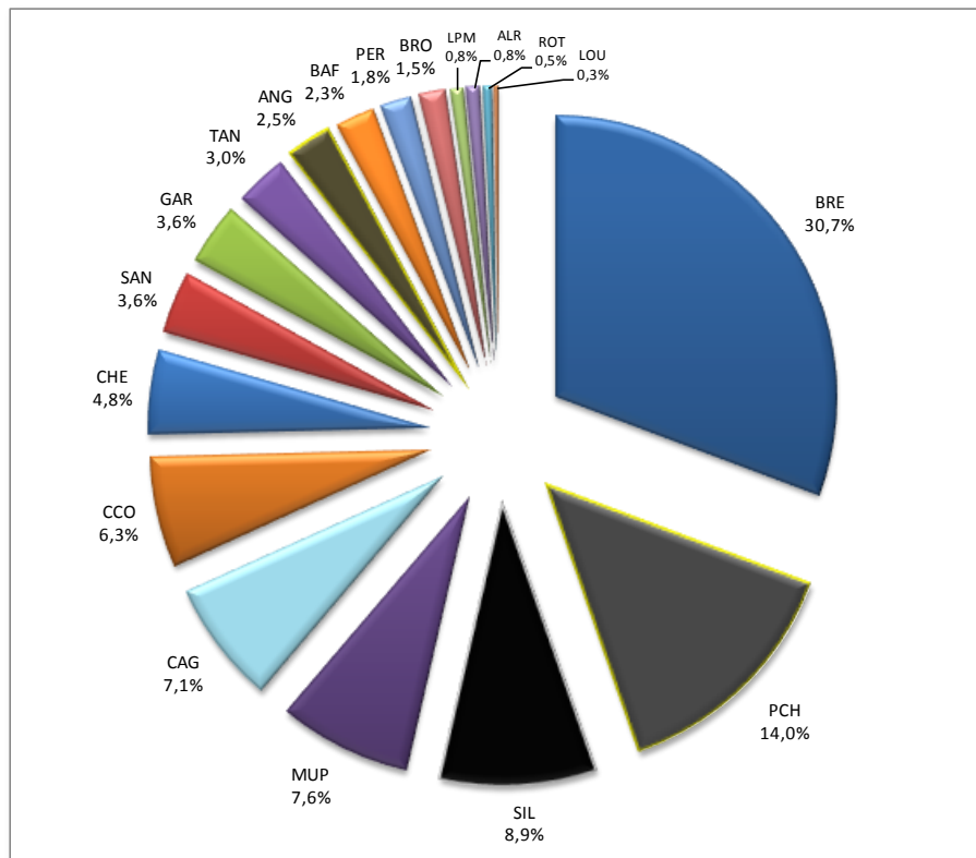
Figure 14: fréquence des espèces piscicoles dans les contenus stomacaux du silure du bassin du Rhône (codes espèces : cf. annexe 3)
