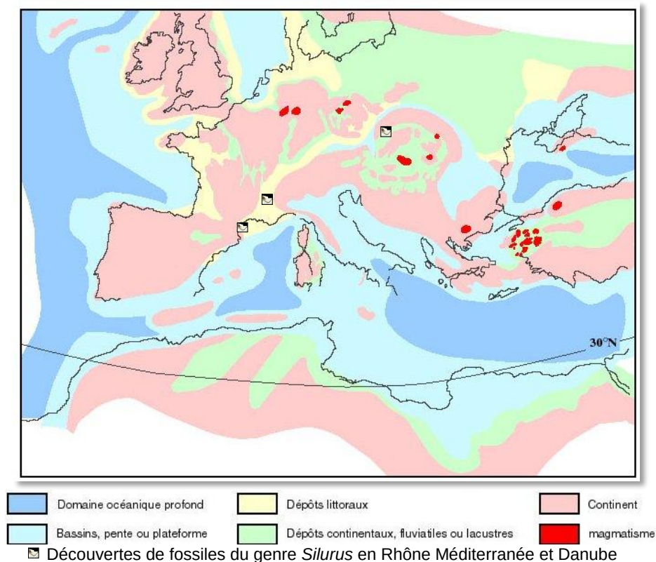
Figure 2 : L'Europe au Miocène moyen (10,5 Ma) et localisation des découvertes de fossiles de silures des bassins méditerranéen et danubien (Carte modifiée d'après Pl. XII in Yilmaz P.O., Norton I., Leary D. et Chuchla R.J. (1996) ; source : http://geologie.mnhn.fr/cenozoique.html )
