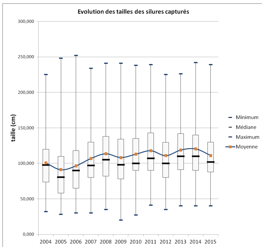
Figure 23 : évolution interannuelle des tailles des silures capturés entre 2004 et 2015
