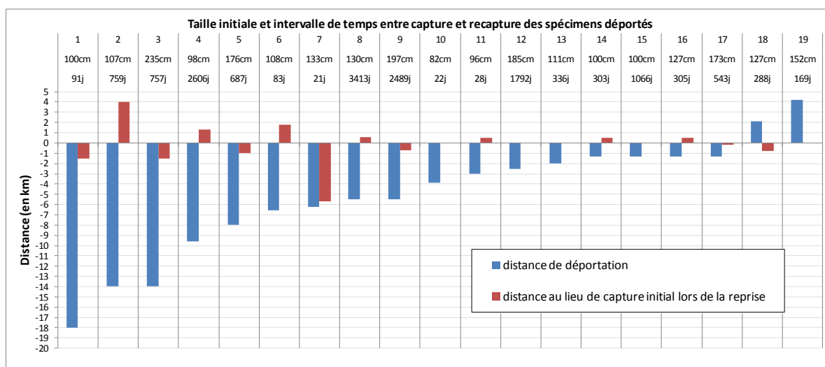
Figure 28 : déplacements effectués par les silures marqués et déportés au cours de cette étude (valeurs négatives : aval, valeurs positives : amont)
