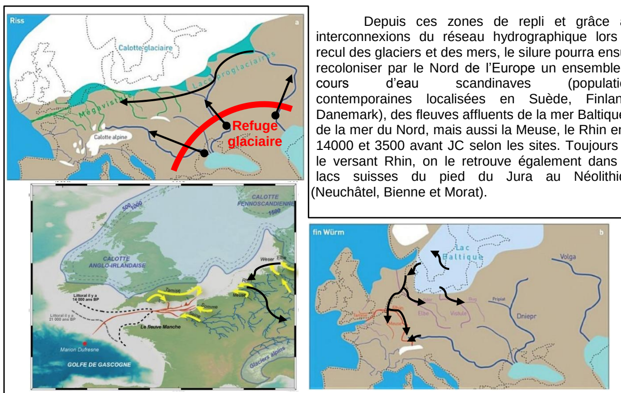
Figure 4 : schématisation des voies probablement empruntées par le silure (flèches noires) pour recoloniser l'Europe de l'Ouest au cours de l'Holocène ; situation du continent eurasiatique au dernier maximum glaciaire : le tracé des côtes à 15 000 et 21 000 ans est illustré par les lignes en pointillés (d'après Persat et Keith, 2011 ; http://www.insu.cnrs.fr/ ).
