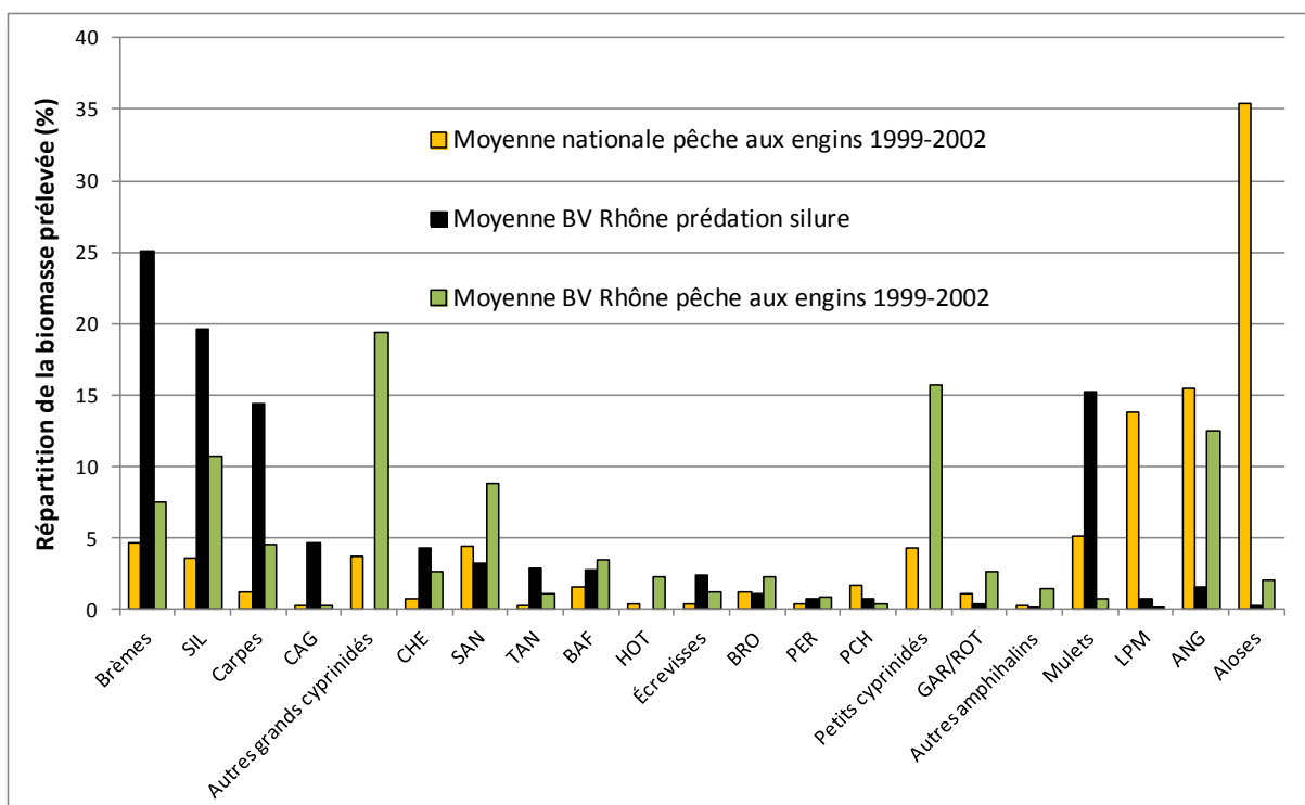
Figure 35 : Répartition du taux de prélèvement de biomasse exercé par la pêche aux engins et par le silure sur les différentes espèces piscicoles (sources : présente étude ; Changeux, 2005 in Keith et al, 2011)
