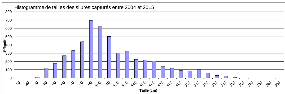
Figure 21 : histogramme des tailles des silures capturés entre 2004 et 2015
