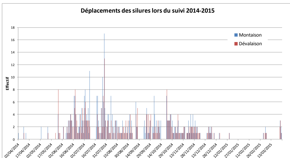
Figure 31 : activité saisonnière des silures observés à la station de vidéo-comptage de Jons
