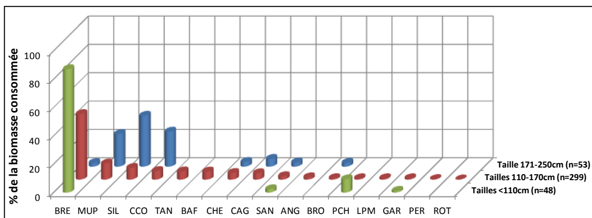
Figure 18 : biomasse des espèces piscicoles dans les contenus stomacaux en fonction de la taille des silures
