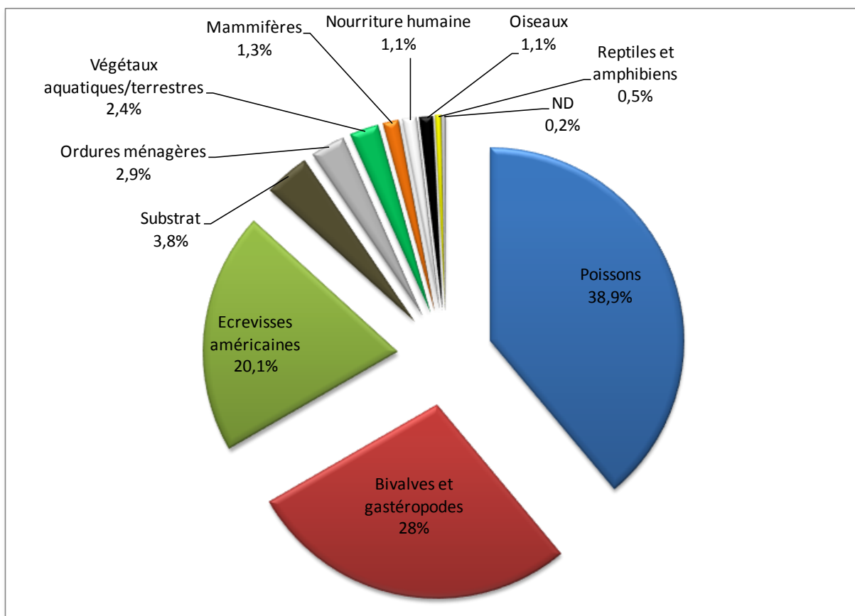
Figure 12 : composition du régime alimentaire du silure du bassin du Rhône (fréquence des éléments dans les contenus stomacaux)
