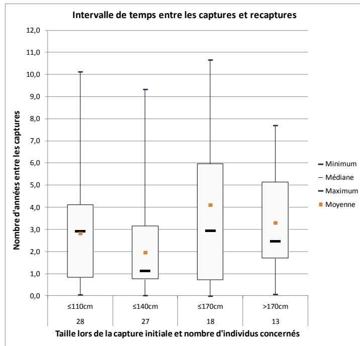
Figure 26 : Caractéristiques temporelles des recaptures selon les classes de taille marquées
