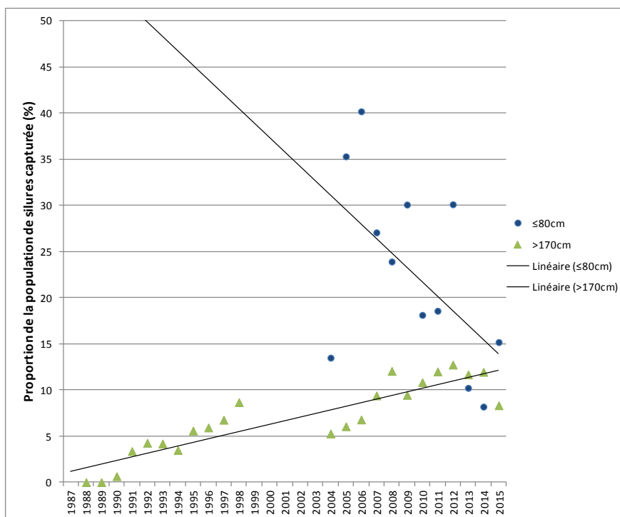
Figure 24 : Evolution des proportions de grands (1987-2015) et petits (2004-2015) silures au sein des populations capturées du bassin du Rhône
