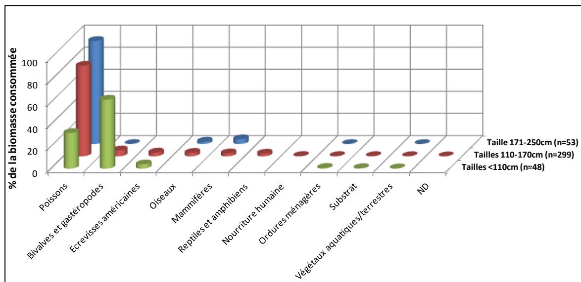
Figure 17 : composition du régime alimentaire du silure du bassin du Rhône (biomasse des éléments dans les contenus stomacaux) en fonction de la taille des poissons
