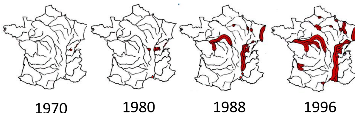
Figure 6 : représentation schématique de la recolonisation du bassin du Rhône et du réseau hydrographique français par le silure ; d'après Tixier, 1998, modifié.
