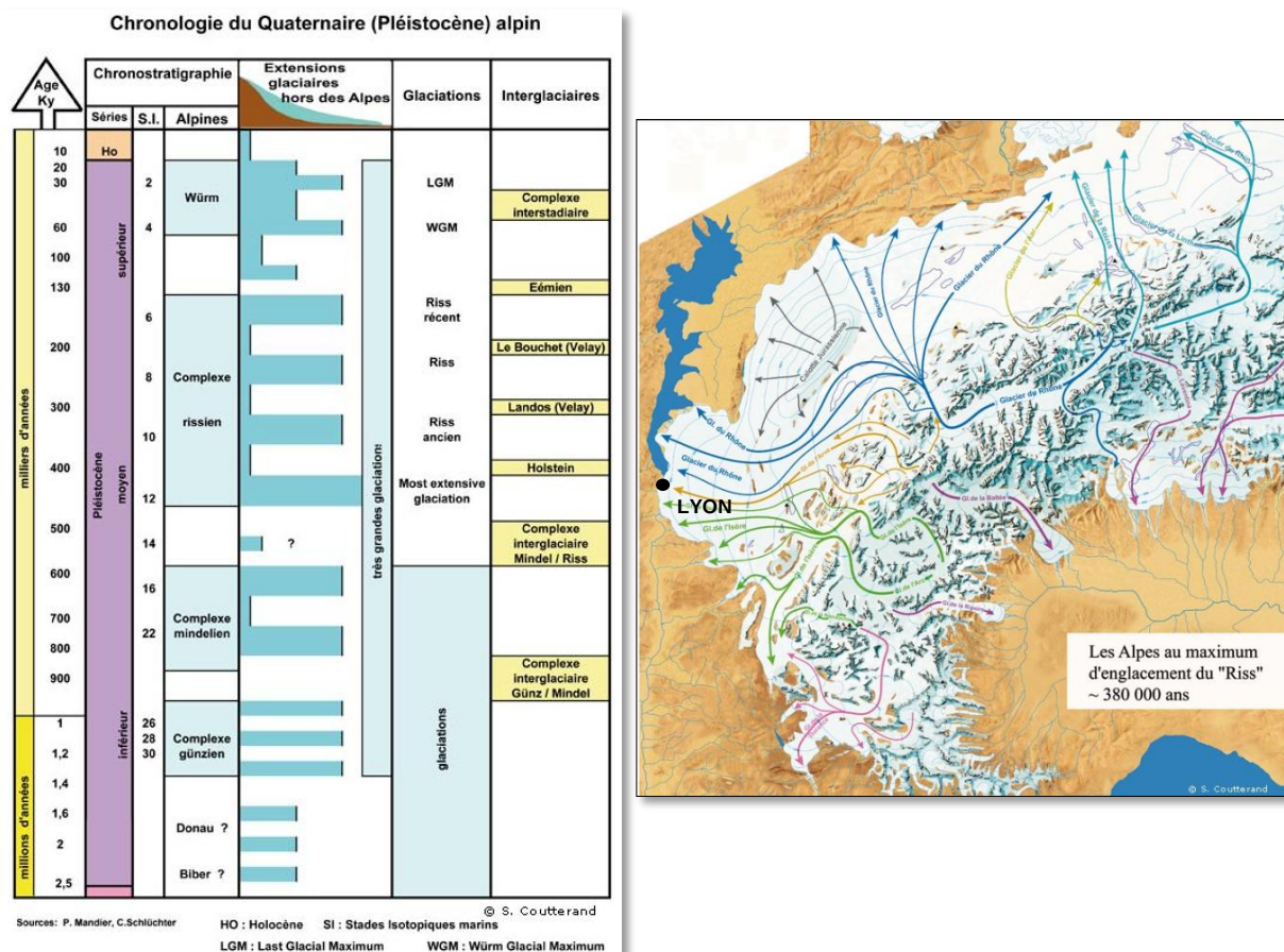
Figure 3 : glaciations et extension des glaciers alpins au cours du temps (source : http://www.glaciers-climat.com/ )
