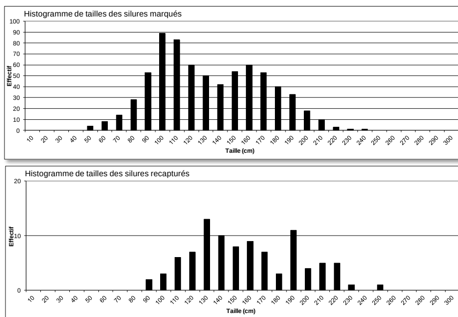
Figure 25 : Histogramme de tailles des silures marqués et recapturés au cours de cette étude
