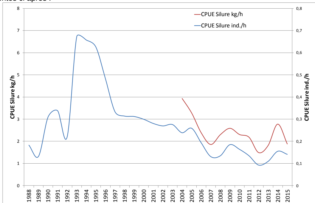
Figure 9 : évolution des CPUE silure sur le grand bassin versant du Rhône entre 1988 et 2015
