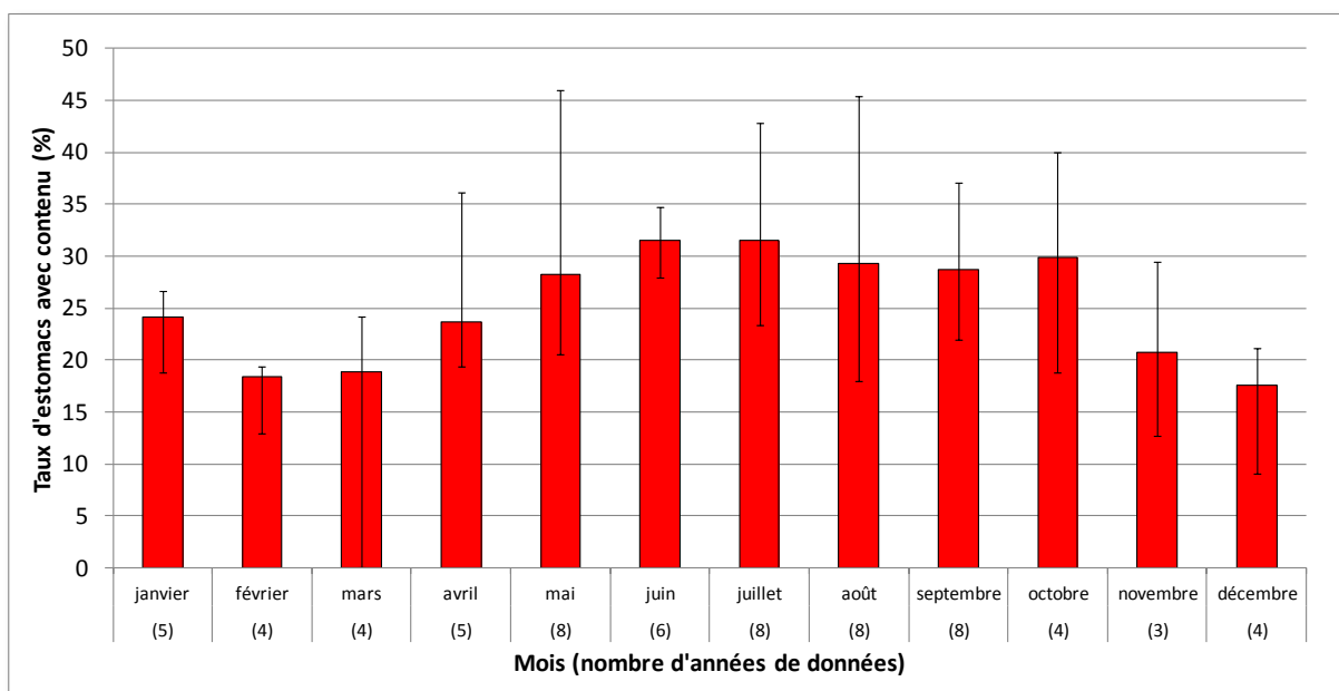
Figure 11 : activité alimentaire mensuelle moyenne du silure dans le bassin du Rhône (avec valeurs minimales et maximales)
