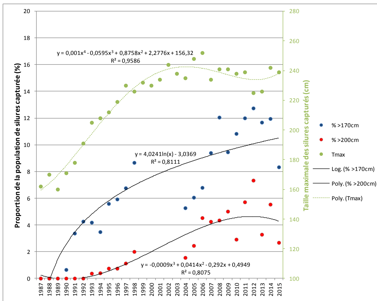
Figure 22 : Evolution des tailles maximales atteintes et de la proportion de grands silures au sein des populations du bassin du Rhône de 1987 à 2015
