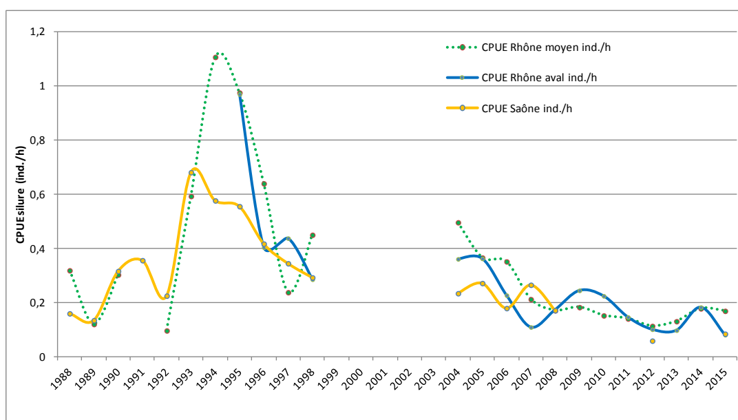
Figure 10 : évolution des CPUE silure par grand secteur de pêche entre 1988 et 2015
