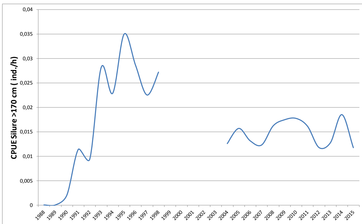
Figure 34 : Evolution des CPUE de silures de tailles supérieures à 170cm dans le bassin du Rhône
