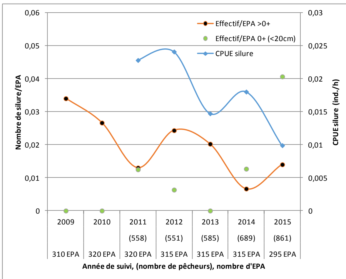
Figure 8 : évolution interannuelle des captures de silure par pêche électrique (6 stations ; FDAAPPMA69 et LEHNA, Université Lyon I) et par pêche à la ligne (3 secteurs ; FDAAPPMA69) sur le Rhône et la Saône dans leur traversée du département du Rhône (cf. carte 1).
