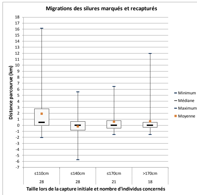
Figure 27 : caractéristiques des déplacements effectués par les silures recapturés au cours de cette étude (valeurs négatives : aval, valeurs positives : amont)
