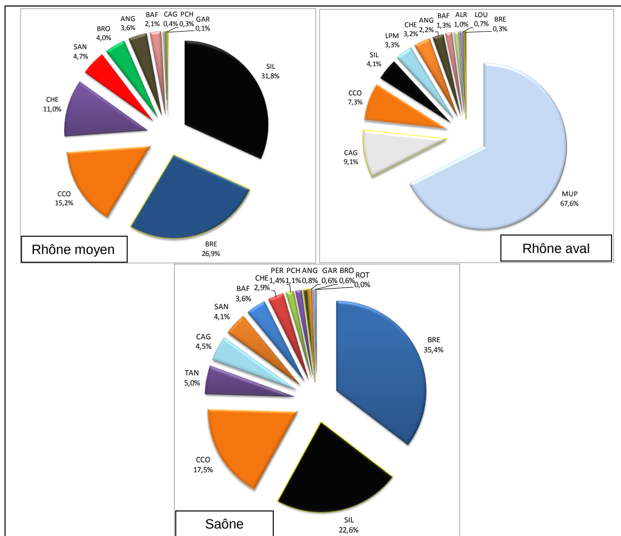
Figure 16 : biomasses respectives estimées des différentes espèces piscicoles observées dans les contenus stomacaux des silures du bassin du Rhône par secteur (codes espèces : cf. annexe 3)
