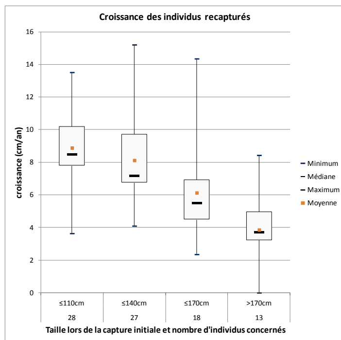
Figure 32 : croissance des silures en fonction de la taille des spécimens calculée à partir des données de marquage/recapture
