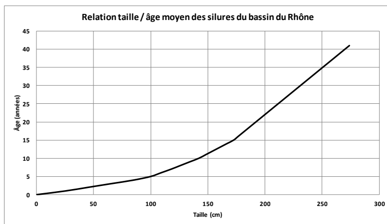
Figure 33 : relation âge-taille des silures du bassin du Rhône
