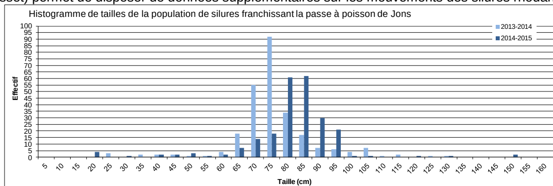
Figure 29 : tailles des silures migrants observés à la station de vidéo-comptage de Jons
