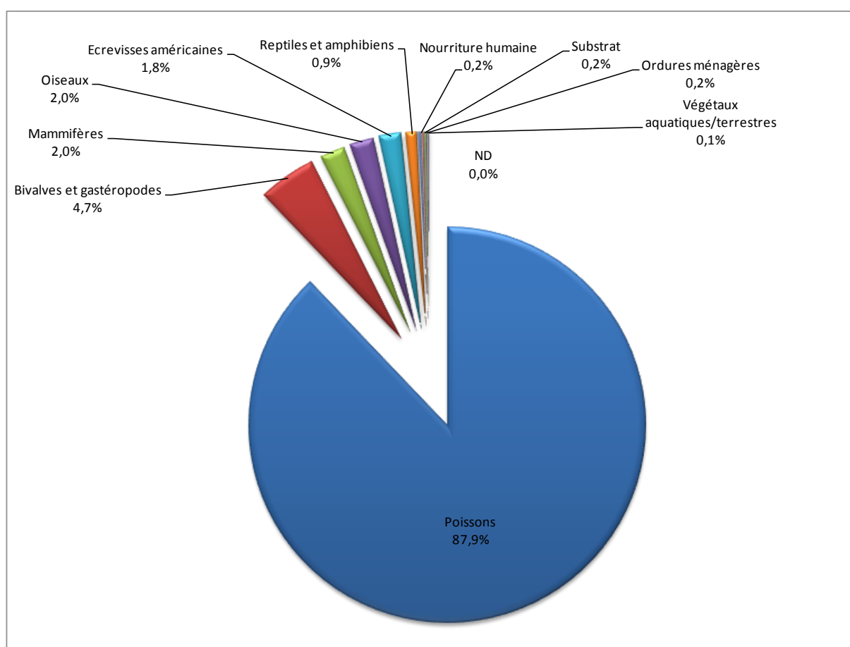
Figure 15: biomasses respectives estimées des différents éléments observés dans les contenus stomacaux des silures du bassin du Rhône
