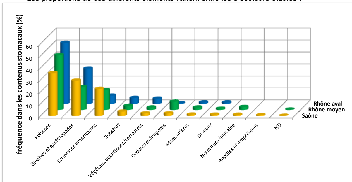
Figure 13 : composition du régime alimentaire du silure du bassin du Rhône (fréquence des éléments dans les contenus stomacaux) en fonction des secteurs
