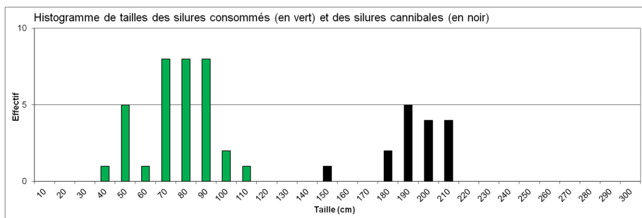
Figure 19 : histogramme de tailles des silures ingérés et de leurs prédateurs
